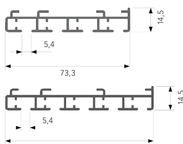
skenprofil 4 & 5 spår
