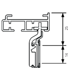
skenprofil med panelvagn
