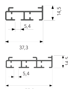
skenprofil 2 & 3 spår
